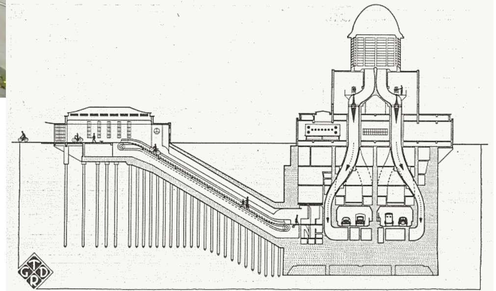
Fig. 15. Doorsnede door ventilatiegebouw, roltrappenschacht en toegangsgebouw.
